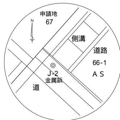
準拠点 J-2詳細図
