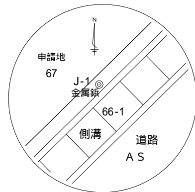
準拠点 J-1詳細図
